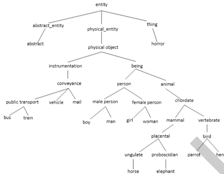
ภาพที่ 3.3 ตัวอย่างจำลอง Synset ในอนุกรมวิธาน WordNet
