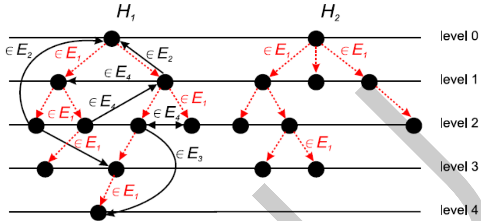
ภาพที่ 3.17 ตัวอย่างการแทนความสัมพันธ์ตามแนวคิดกราฟ
