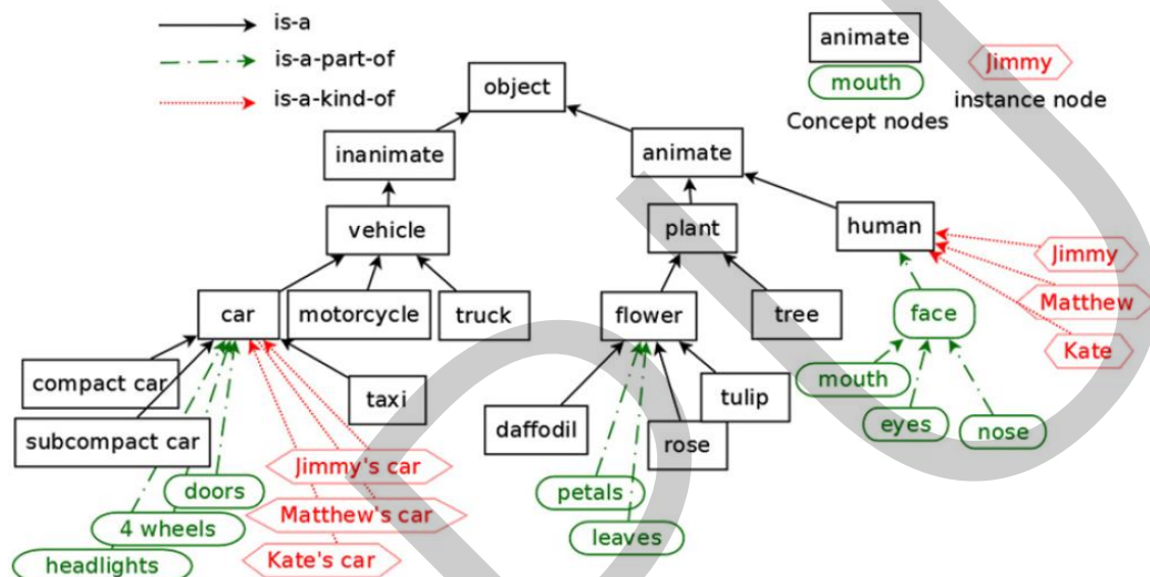
ภาพที่ 2.6 ตัวอย่างแนวคิดเครือข่ายความสัมพันธ์ระหว่างคำอธิบายความหมายบนภาพ
